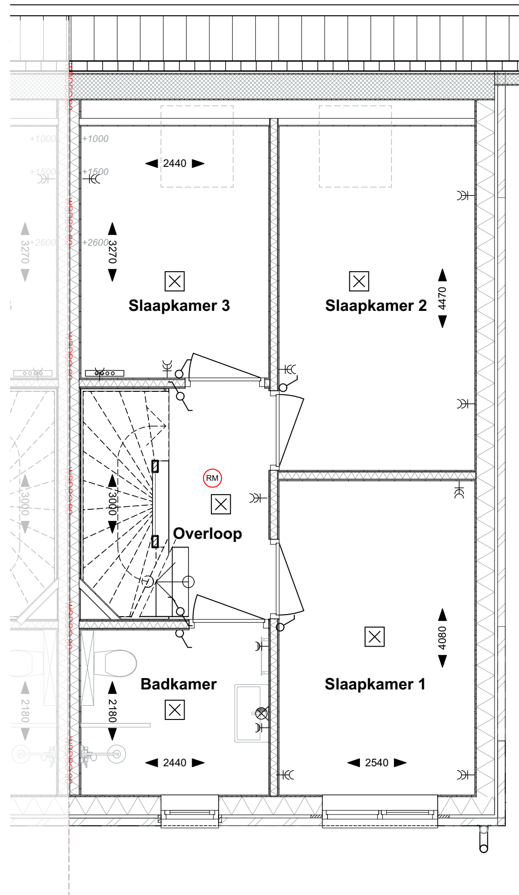
1e Verdieping
