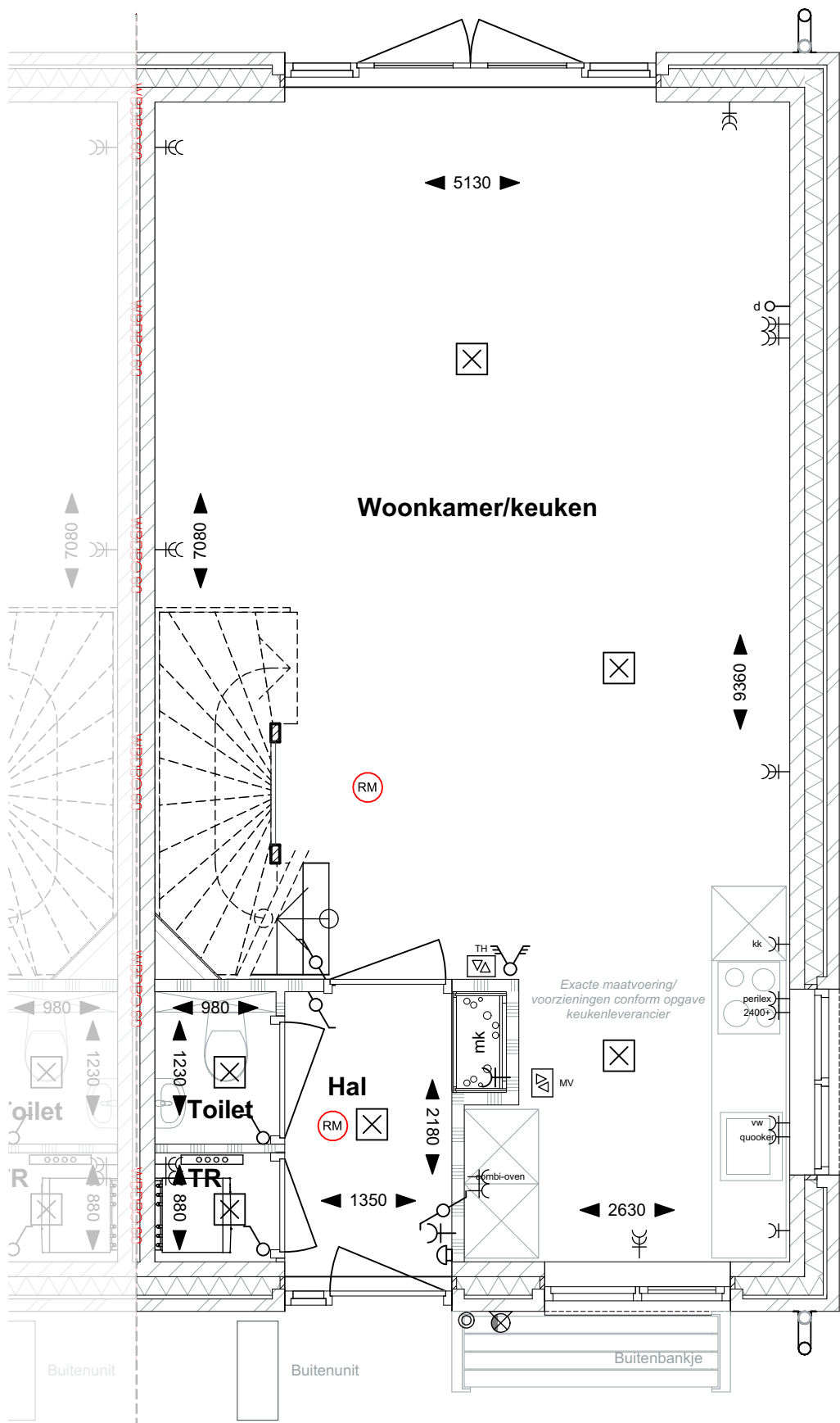
Begane Grond
