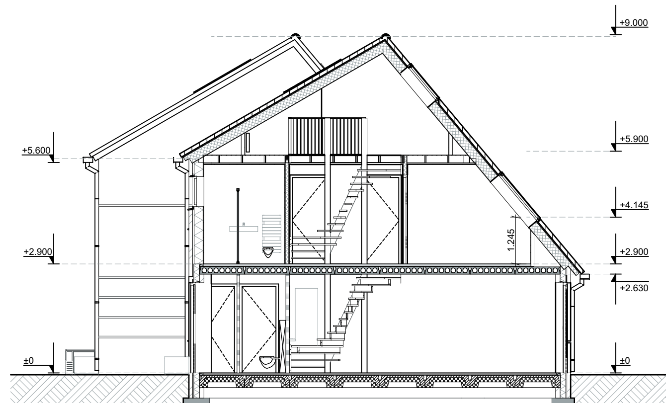
Doorsnede
