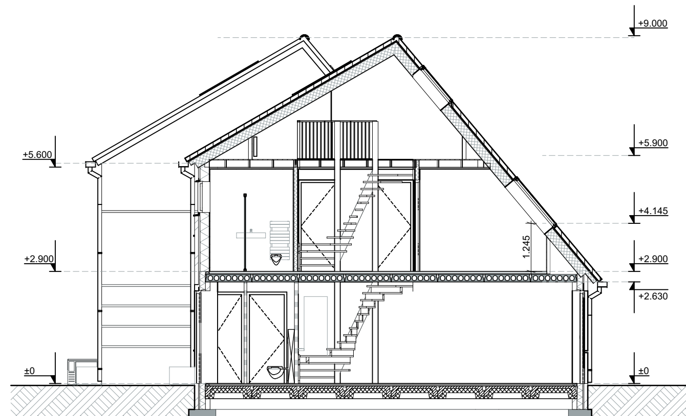
Doorsnede
