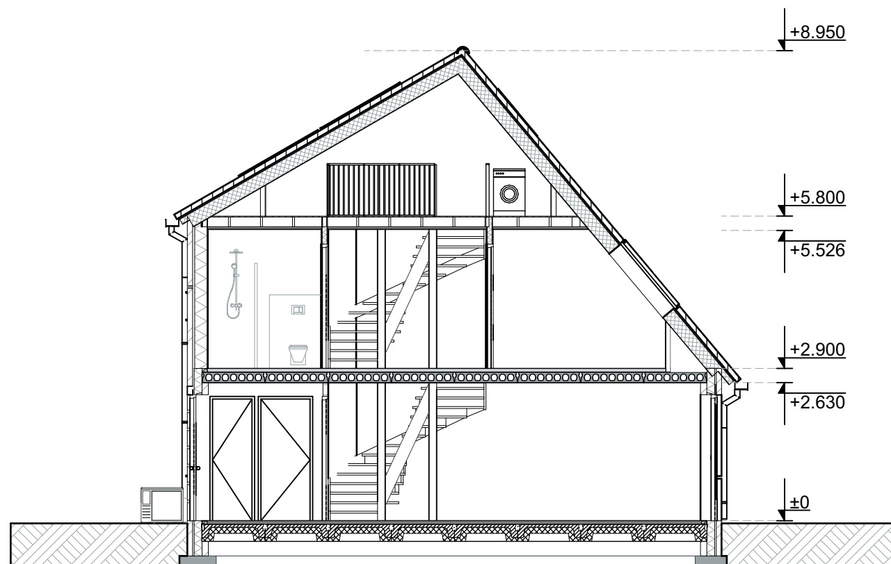
Doorsnede
