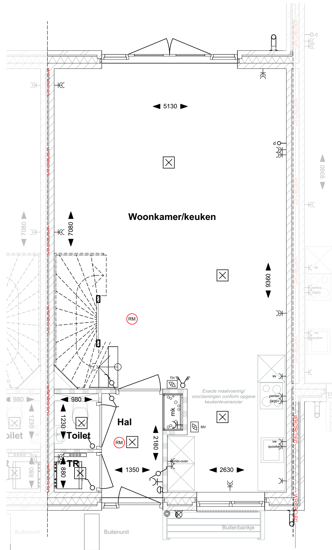
Begane Grond
