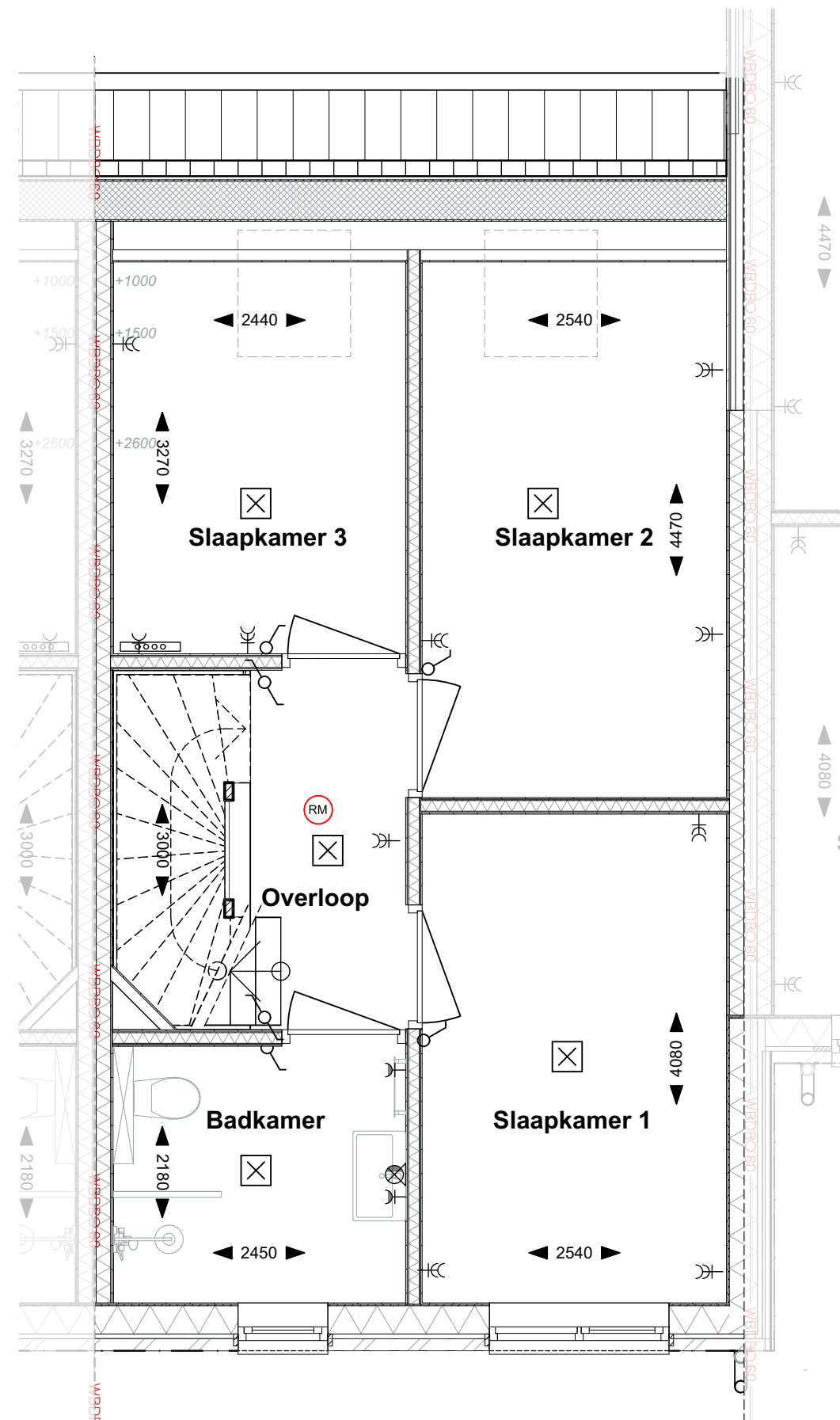
1e Verdieping
