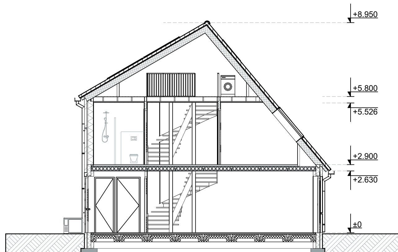
Doorsnede
